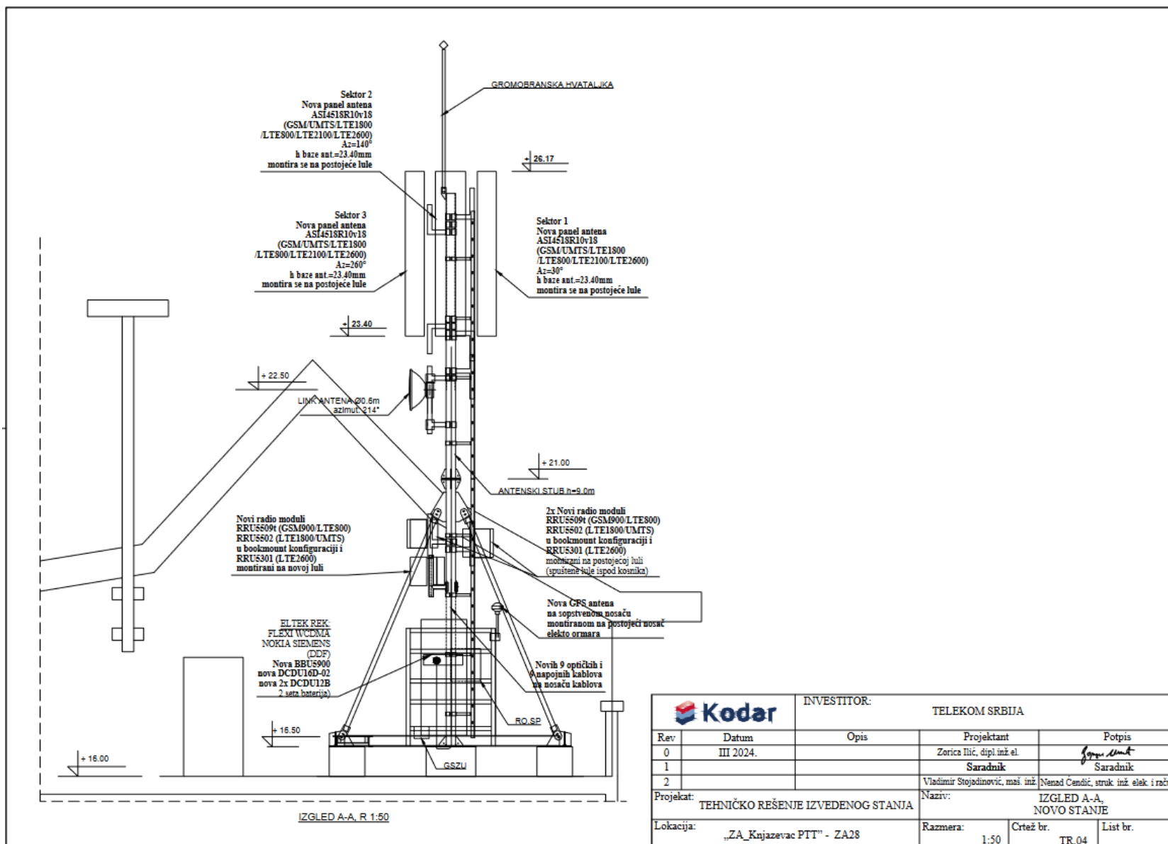
Слика 3.2. Техничко решење изведеног стања – изглед А-А – ново стање
