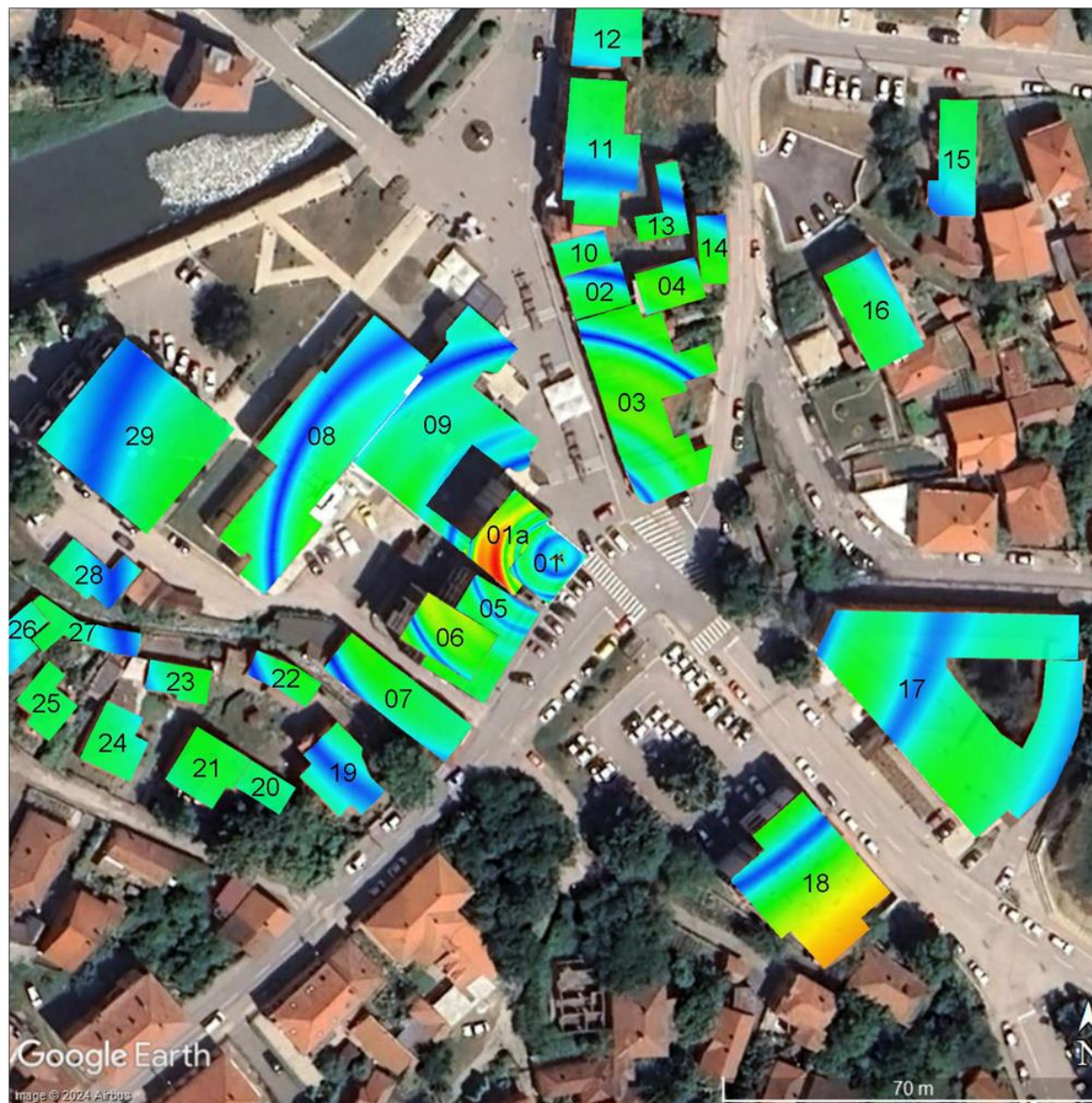
Слика 6.9. Јачина електричног поља унутар објекта када радио-систем UMTS2100 оператора Telekom Srbija ради максималним капацитетом
