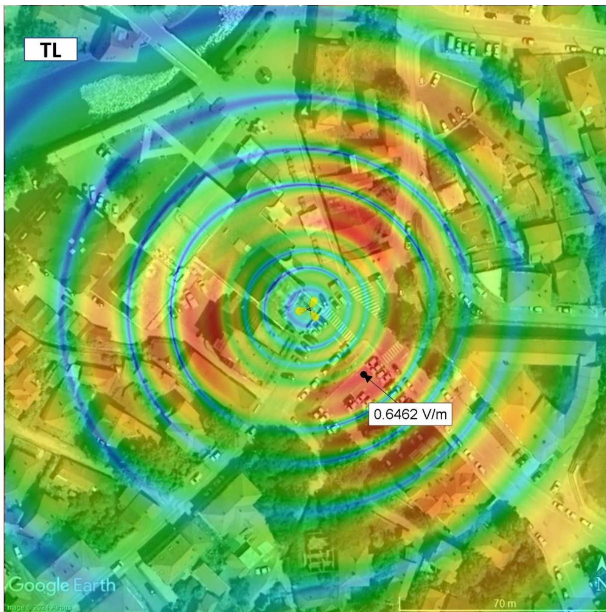
Слика 6.3. Јачина електричног поља на тлу када радио-систем UMTS2100 оператора Telekom Srbija ради максималним капацитетом
