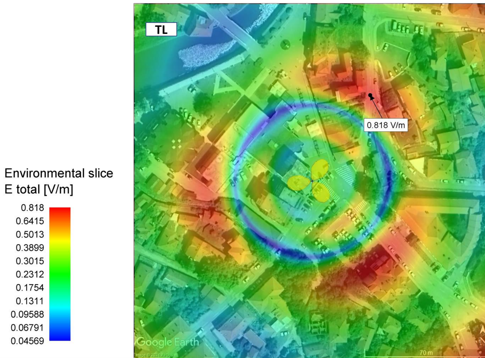
Слика 6.2. Јачина електричног поља на тлу када радио-систем GSM900 оператора Telekom Srbija ради максималним капацитетом
