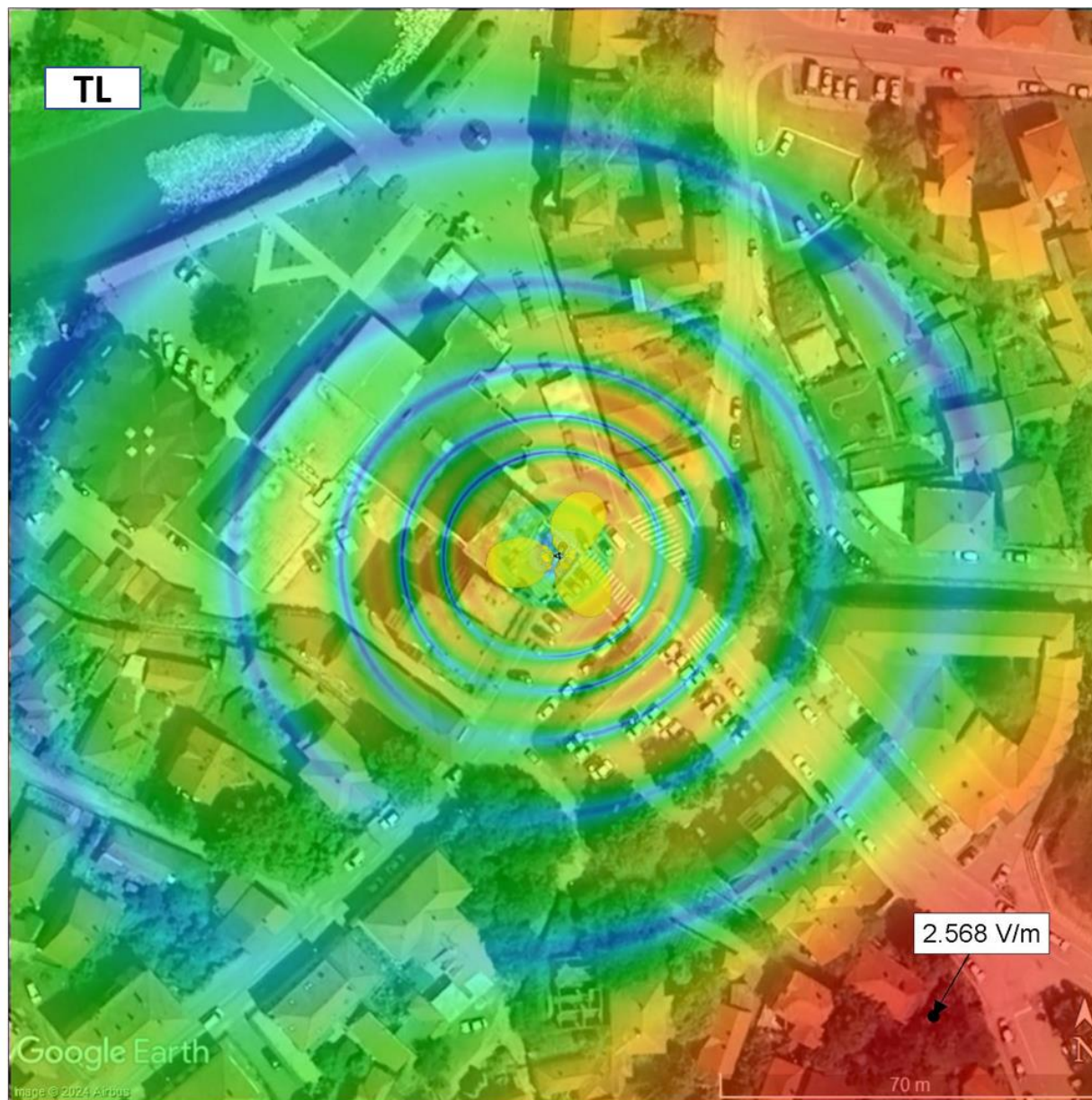
Слика 6.5. Јачина електричног поља на тлу када радио-систем LTE1800 оператора Telekom Srbija ради максималним капацитетом
