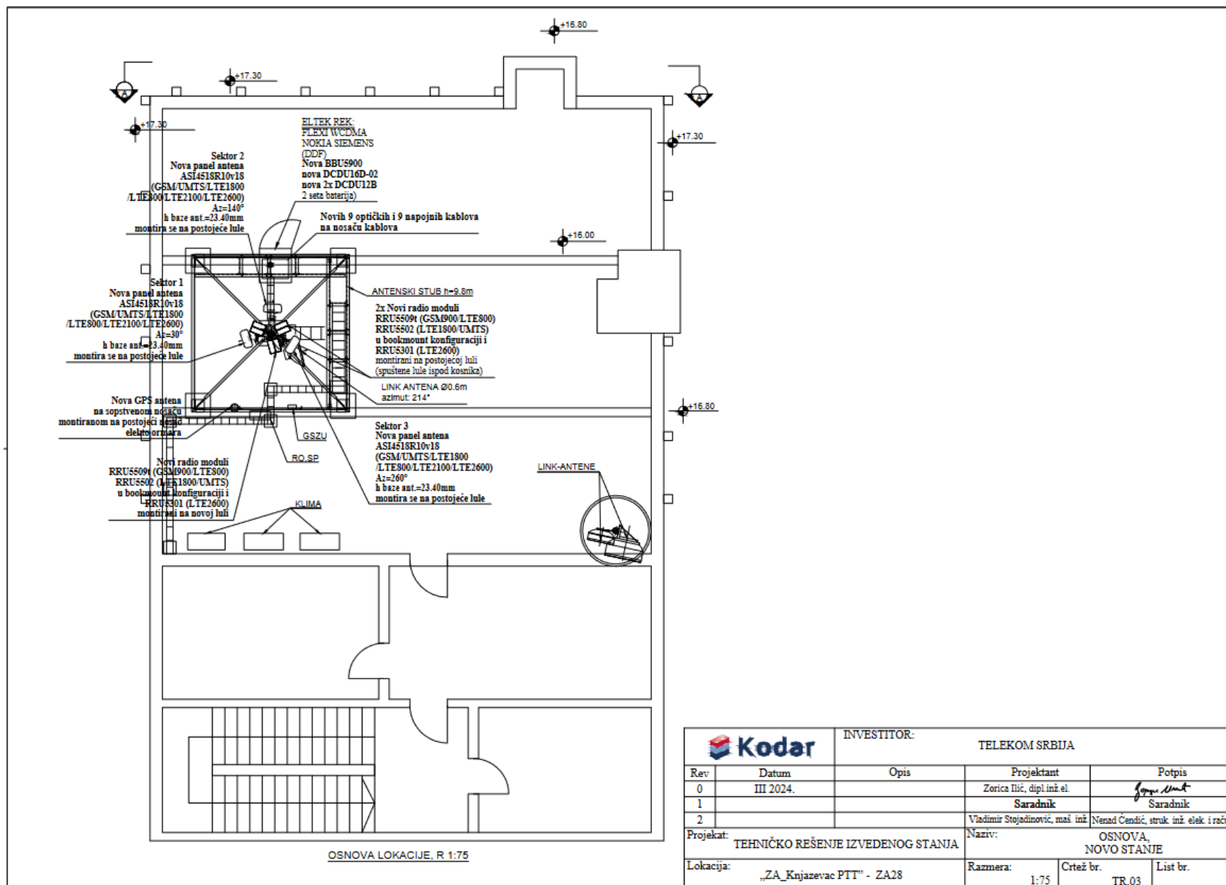
Слика 3.1. Техничко решење изведеног стања – основа – ново стање
