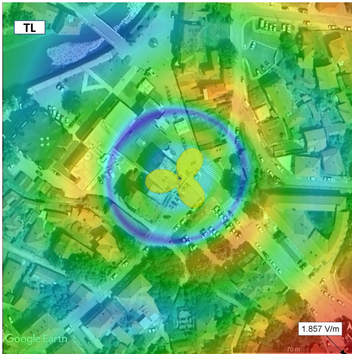
Слика 6.4. Јачина електричног поља на тлу када радио-систем LTE800 оператора Telekom Srbija ради максималним капацитетом
